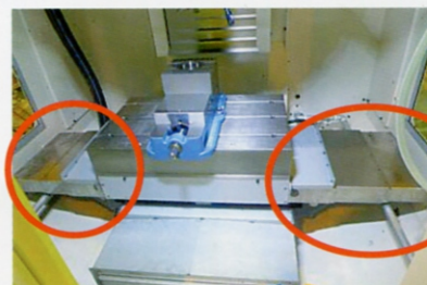
三段式（左右）
