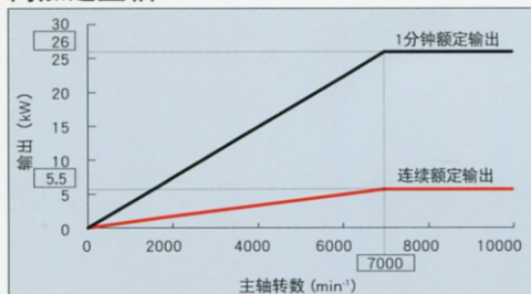
高加速主轴
